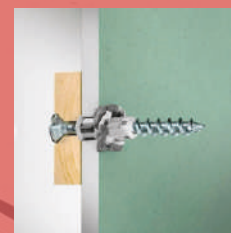
Панельные материалы с шурупом для ДСП
