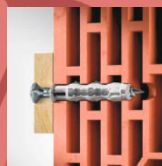
Пустотелый
